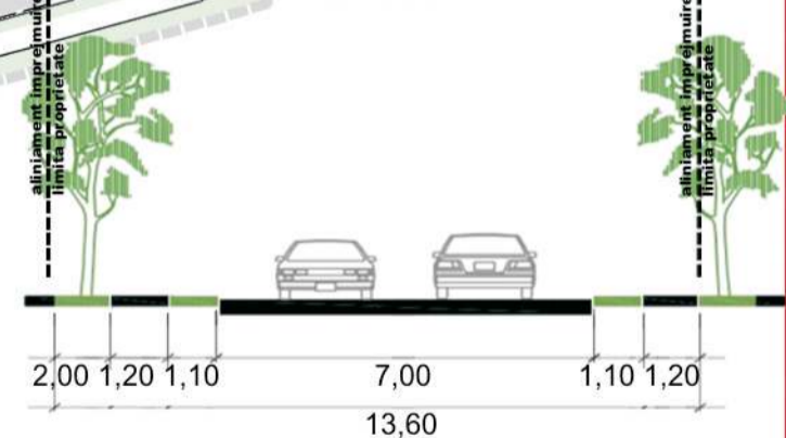
PROFIL STRADA I.C. BRATIANU - existent strada cat a II-a
