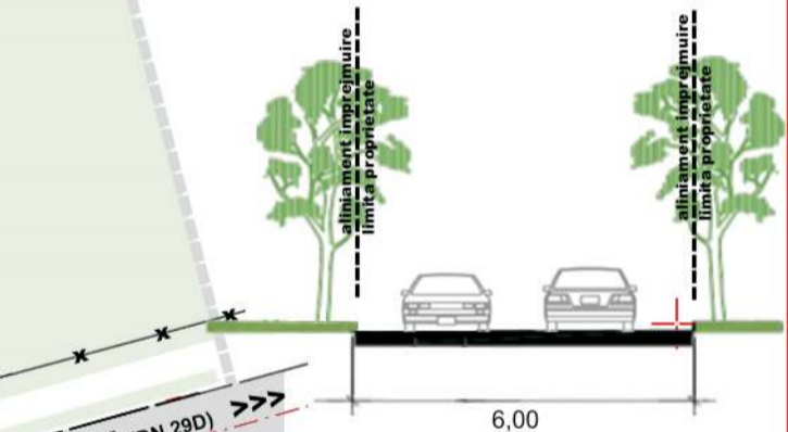
PROFIL ALEE CAROSABILA - propusa strada cat a IV-a - 2 benzi semicarosabil
