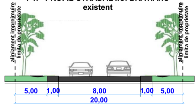
P2 - PROFIL STRADAL D.E.228 existent
